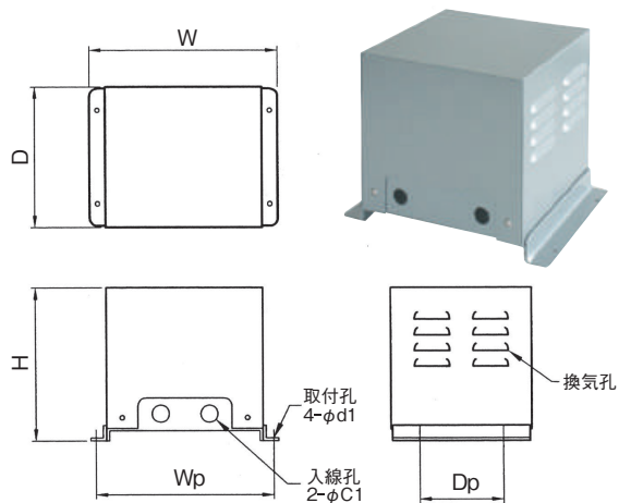
図-A1
