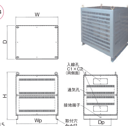
図-A4
