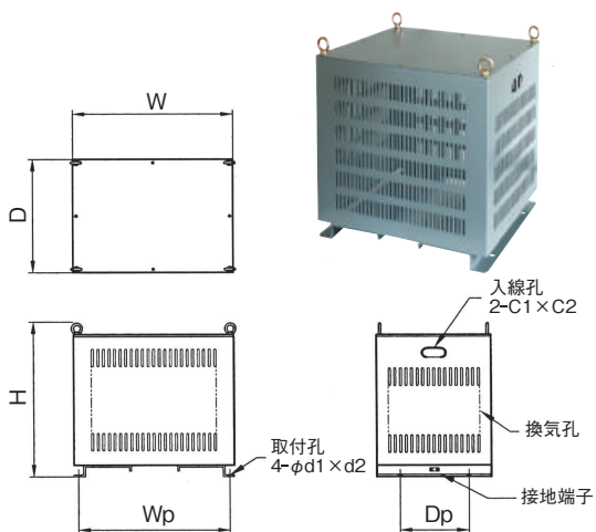
図-A3
