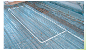
検知器・ループコイル
