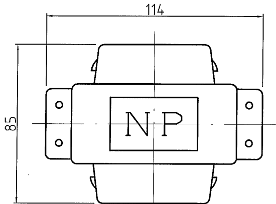
外形図
