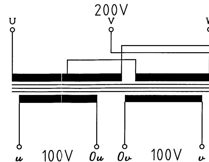
結線図
